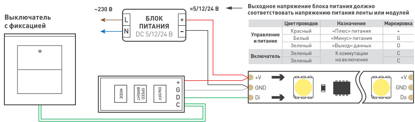
Рис. 1. Подключение одной SPI-ленты с током потребления менее 2 А
